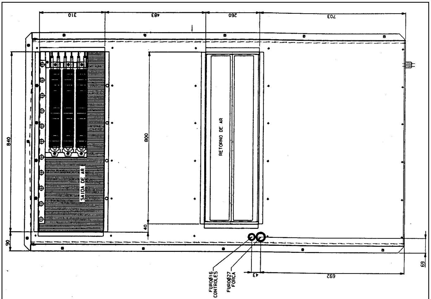
Figura 3a - Dimensões das unidades 50BWF 24/36
